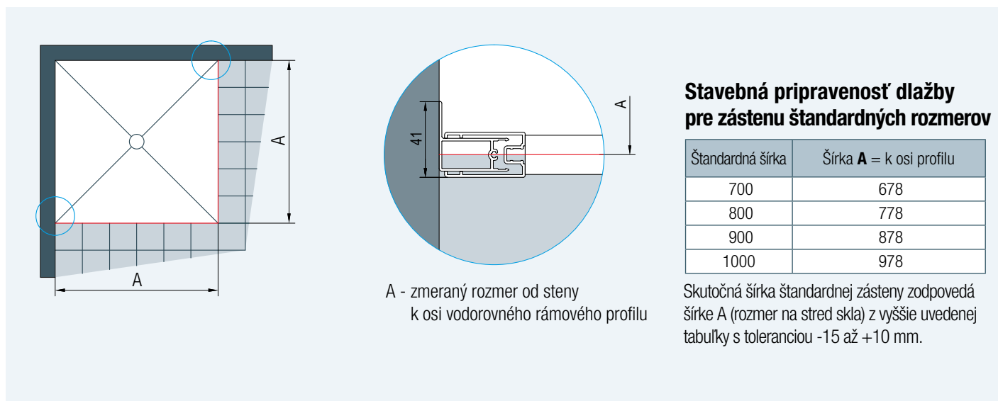
Obr. 2: Pri montáži na dlažbu sa pri výrobe nezohľadňuje žiadne odsadenie.
