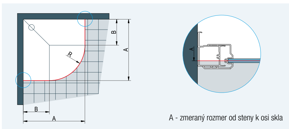
Obr. 4: Pri montáži na dlažbu sa pri výrobe nezohľadňuje žiadne odsadenie. U dlažby je nutné zohľadniť rádius R477 alebo R527 (pozri tabuľky vpravo).
