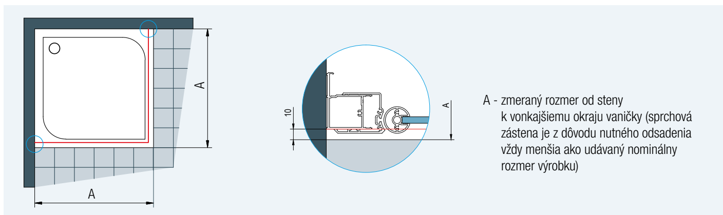
Obr. 1: Pri montáži na vaničku je odsadenie 10 mm rovnaké pre štandardné aj špeciálne rozmery.
