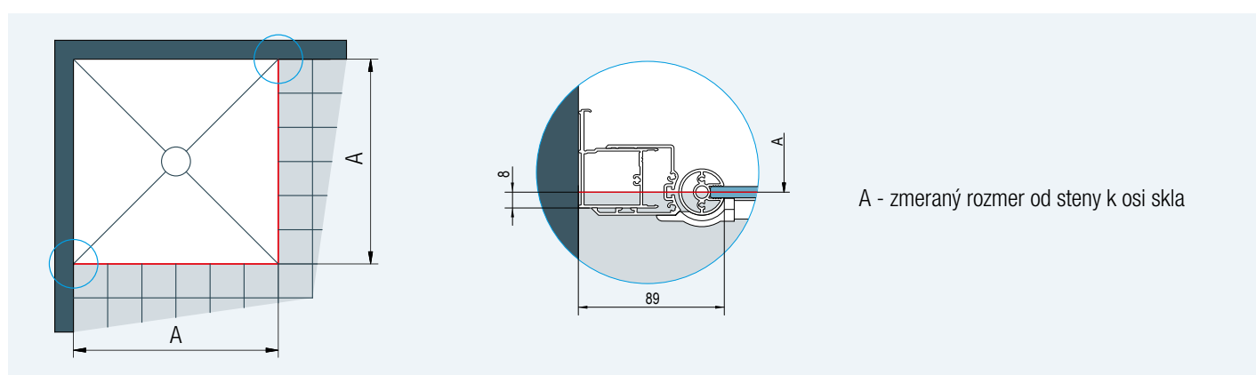
Obr. 2: Pri montáži na dlažbu sa pri výrobe nezohľadňuje žiadne odsadenie
