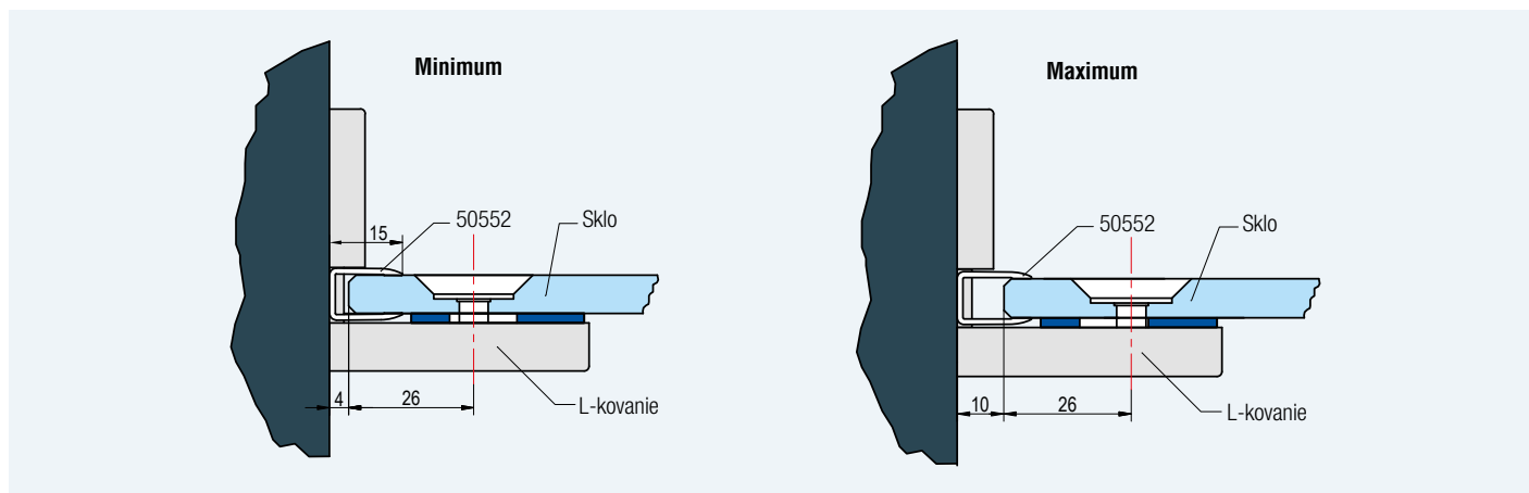
Obr. 5: L-kovanie s tesniacim U-profilom 50552 umožňuje vyrovnanie nerovností steny do 6 mm. Tesniaci U-profil 50552 umožňuje zakryť medzeru medzi stenou a sklom.
