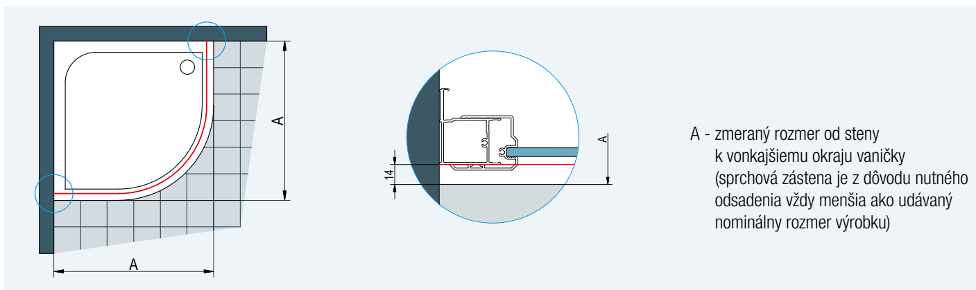
Obr. 3: Pri montáži na vaničku je odsadenie 14 mm rovnaké pre štandardné i zvláštne rozmery
