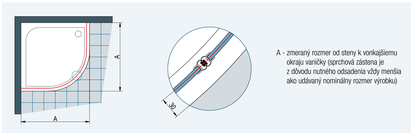
Obr. 3: Pri montáži na vaničku je odsadenie 30 mm rovnaké pre štandardné i zvláštne rozmery.
