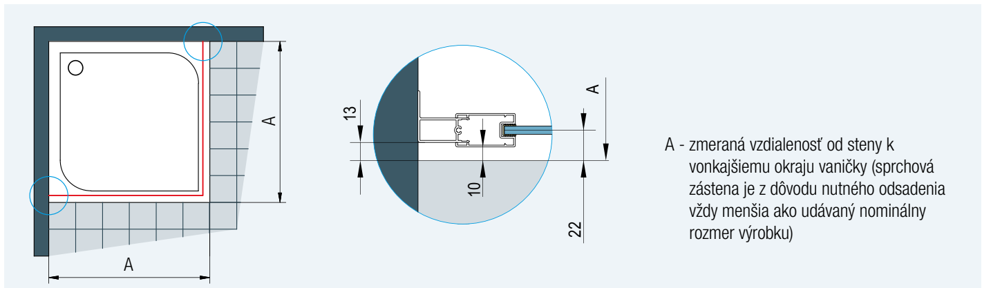
Obr. 1: Pri montáži na vaničku je odsadenie 13 mm rovnaké pre štandardné aj špeciálne rozmery.
