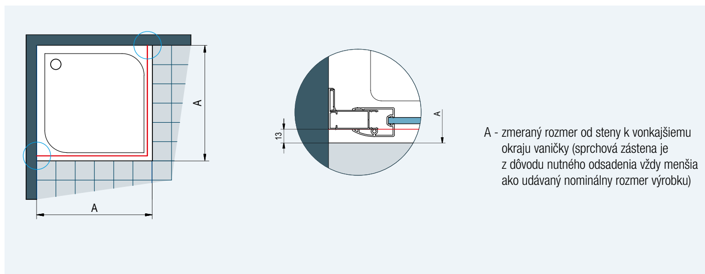
Obr. 1: Pri montáži na vaničku je odsadenie 13 mm rovnaké pre štandardné aj špeciálne rozmery.
