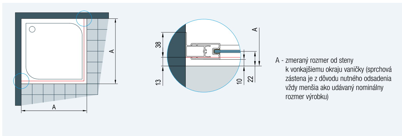
Obr. 1: Pri montáži na vaničku je odsadenie 13 mm.
