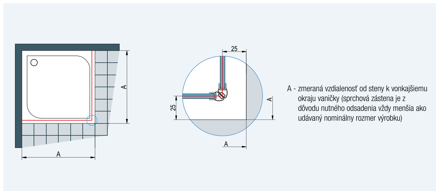
Obr. 1: Pri montáži na vaničku je odsadenie 25 mm rovnaké pre všetky typy série ESCURA.
