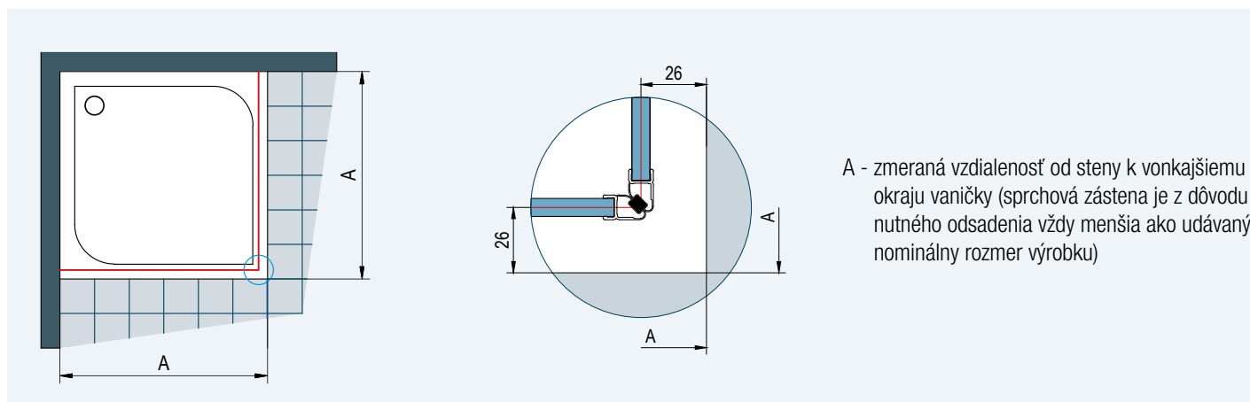
Obr. 1: Pri montáži na vaničku je odsadenie 26 mm rovnaké pre štandardné i zvláštne rozmery.
