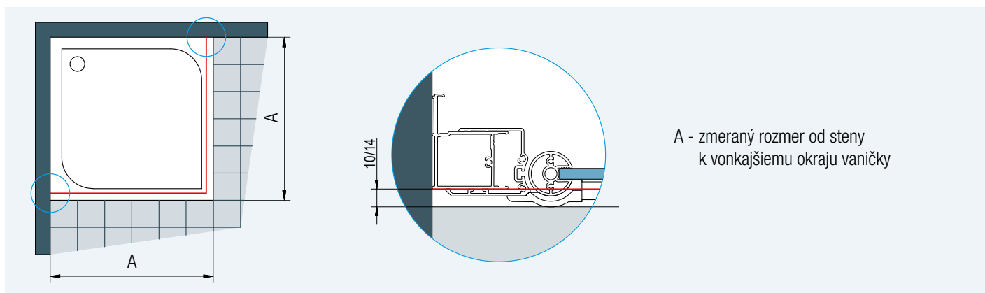
Obr. 1: Pri montáži na vaničku je pri dverách s bočnou stenou odsadenie 10 mm rovnaké pre štandardné aj špeciálne rozmery. U rohového vstupu je odsadenie 14 mm.
